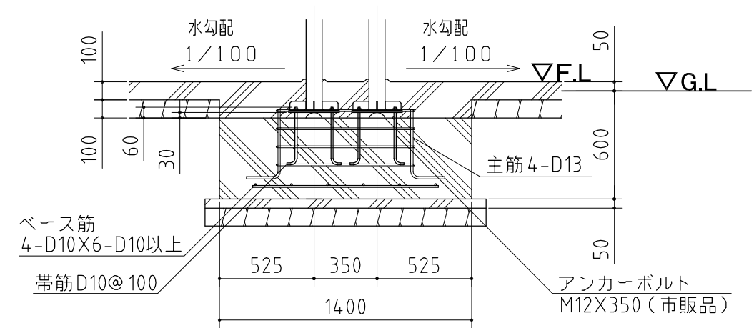
A-A' 断面
